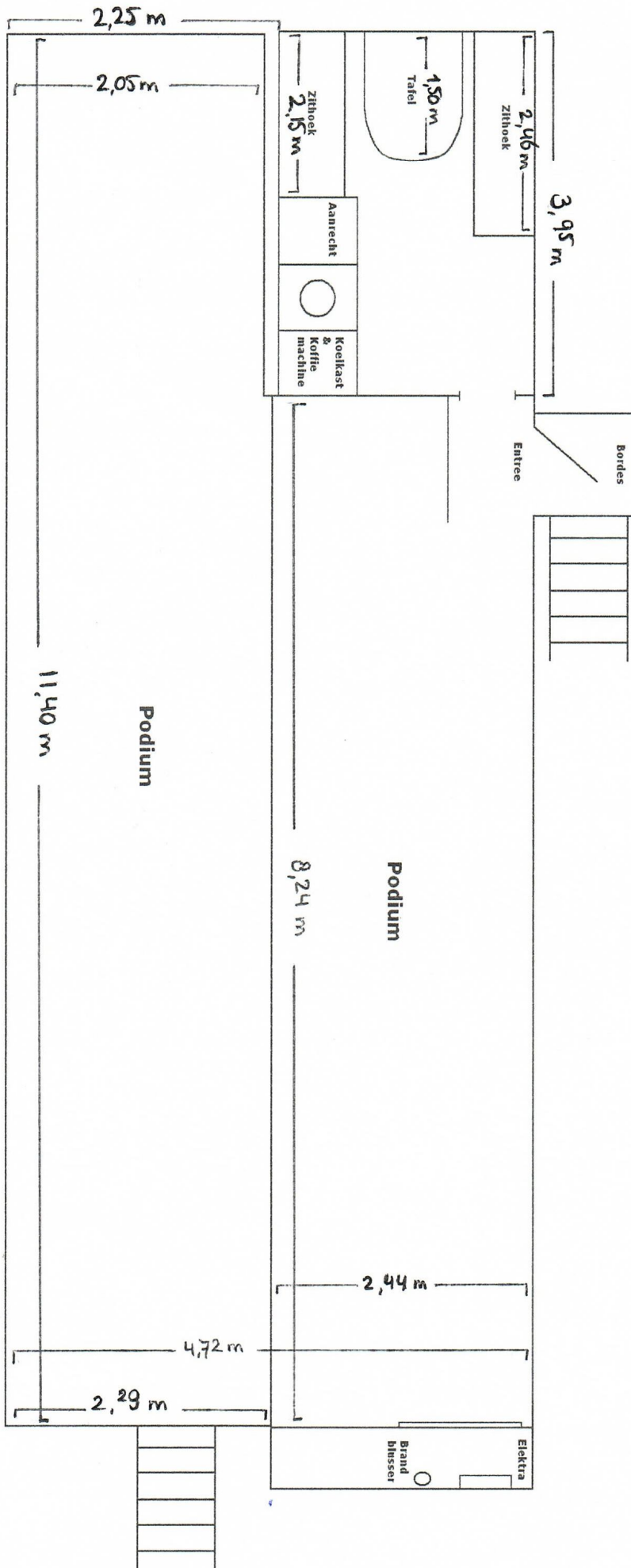
Podiumwagen boven aanzicht
